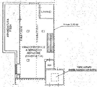
PIANO SOTTOTETTO H = 2,39 ml
